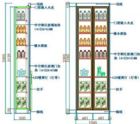
酒柜8剖面图
