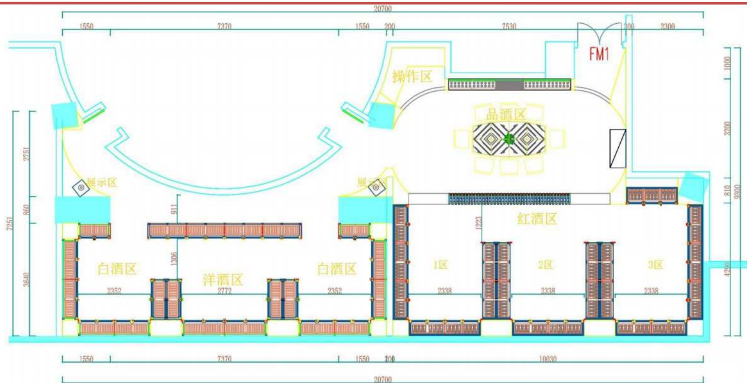
平面布置图
