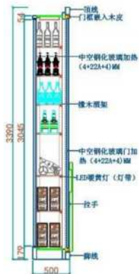
酒柜12剖面图
