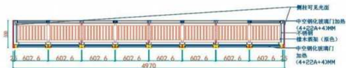
酒柜7平面图
