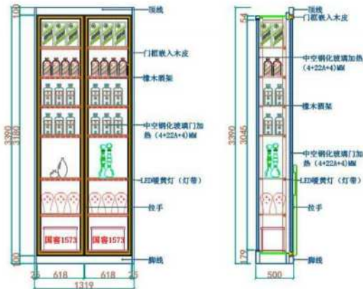
酒柜11立面图
