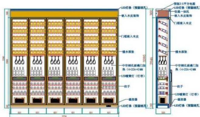
酒柜4立面图
