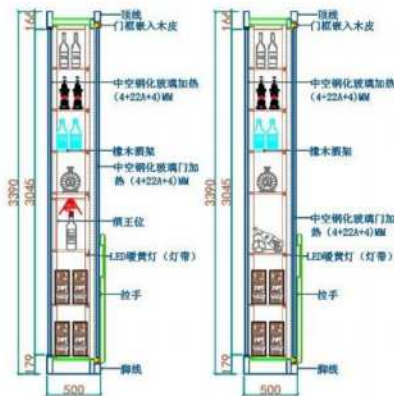
酒柜7剖面图
