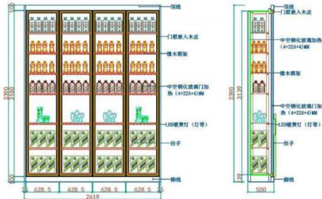
酒柜9立面图
