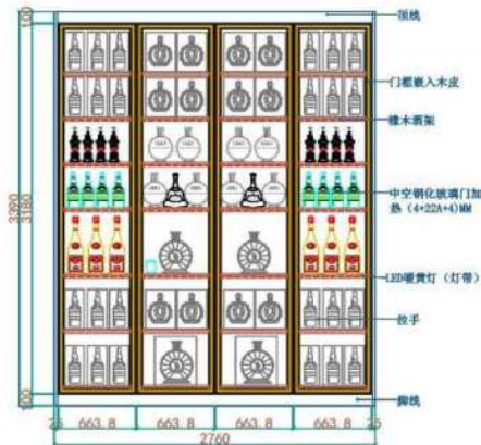
酒柜13立面图
