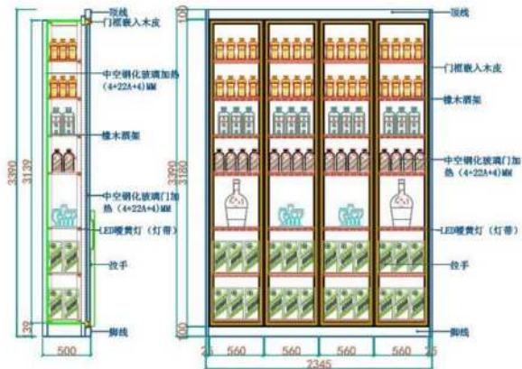
酒柜10剖面图
