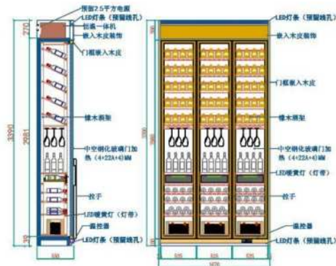
酒柜3剖面图
