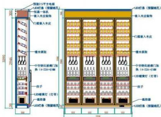
酒柜5剖面图
