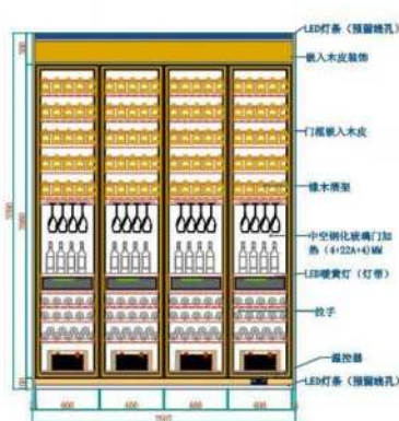
酒柜6立面图
