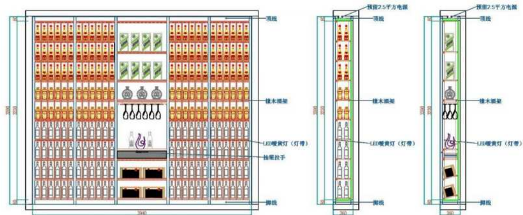
酒架1立面图
