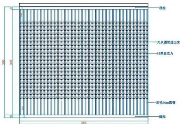
酒架2立面图
